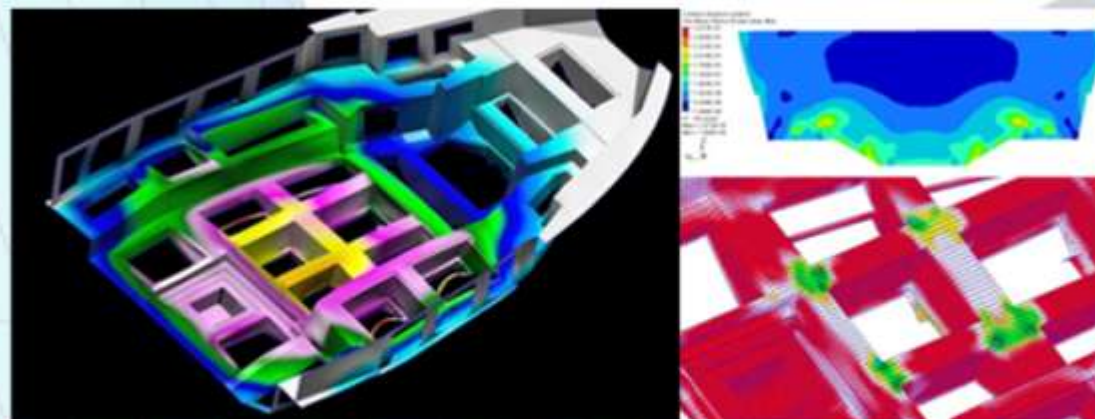
Analisi degli elementi finiti (FEA) su scafo in materiale composito
