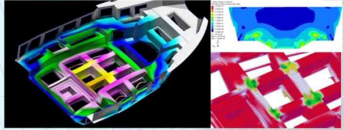
Kompozit gövdede ölçülebilir öge analizleri
