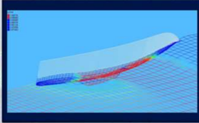
U/UREF-CFD Yelkenli tekne gövdesi simülasyonu
